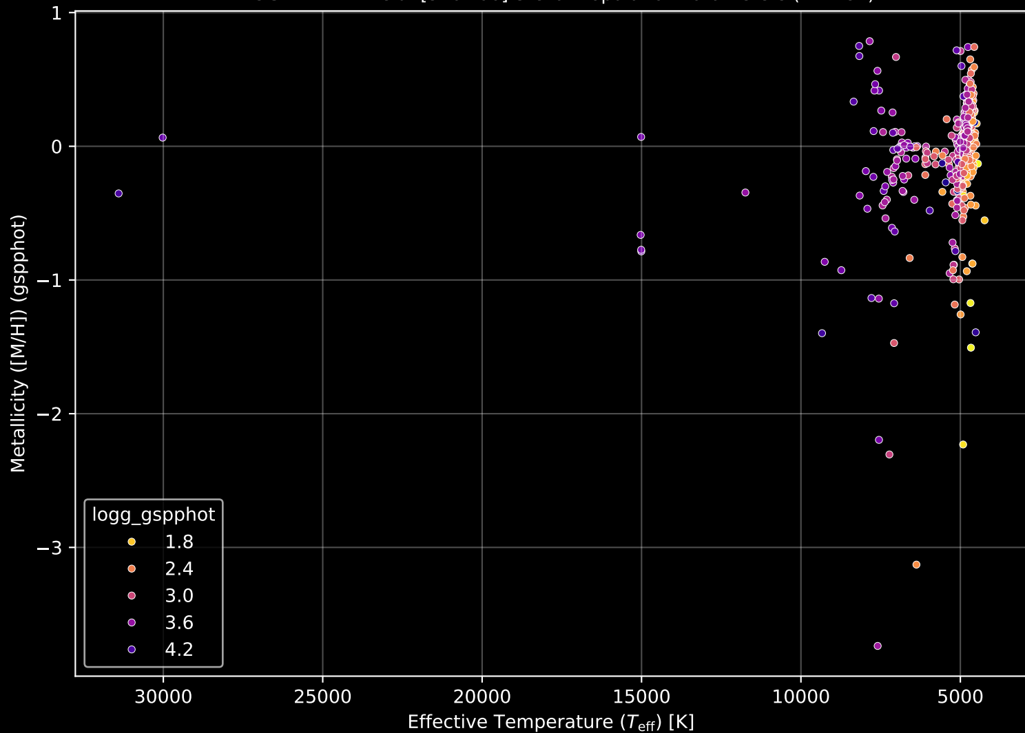
APOGEE DR17 Field: [340+06] Stellar Population Parameters (n= 481)
